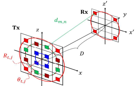
그림 1. 제안하는 Max-Min 채널 용량 전략 기반 부배열 선택 기법의 시스템 모델.
