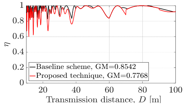
그림 2. LoS MIMO 환경에서 제안하는 기법의 채널 용량 이득 성능. 거리에 대한 GM은 그림 2와 같고 구간별 GM은 표 1과 같다. 제안하는 기법은 모든 전송 거리에 대해 안테나 배치 최적화를 수행한 기존 기법 대비 평균 0.0968 정도의 구간별 GM 오차를 갖는 것을 확인하였다. 따라서, 제안하는 기법은 주어진 구간에 대해 동일한 부배열로 통신하더라도 우수한 공간 다중화 성능을 보이므로 실제적인 LoS MIMO 통신시스템 운용 방안으로 활용될 수 있다.
